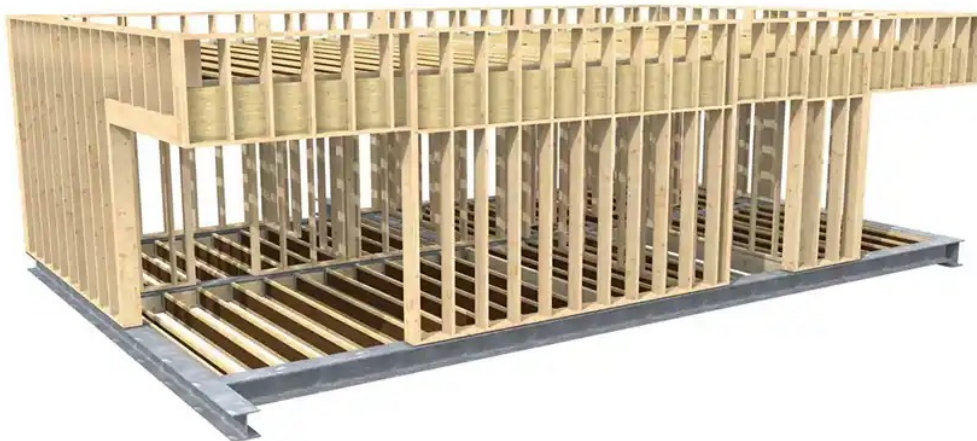
Eco Kit · model van de houtstructuur uit KiteHouse-projectmateriaal
